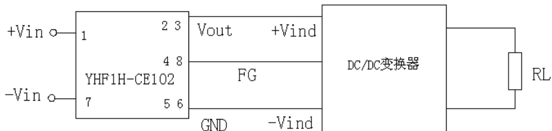
图 3 典型应用图
