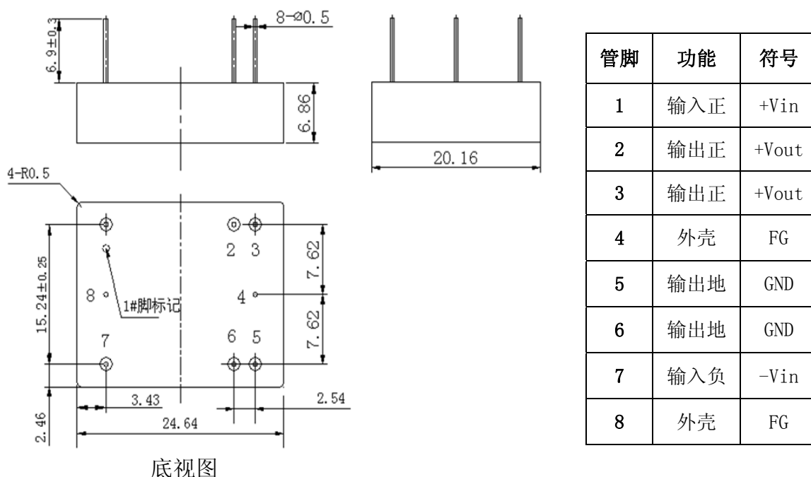
图 1 外形尺寸及引脚功能
