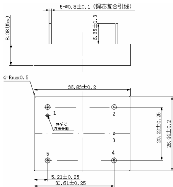
底视图
