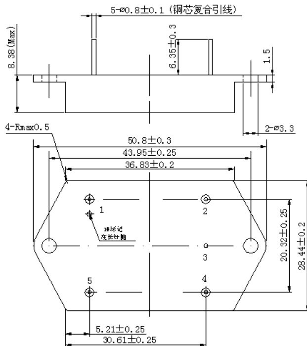
底视图
