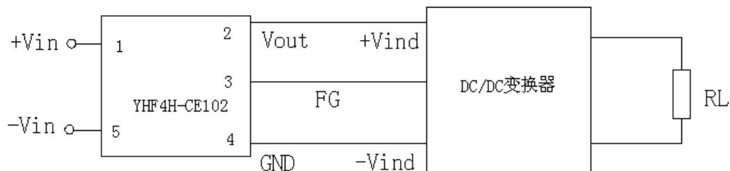
图 3 典型应用图
