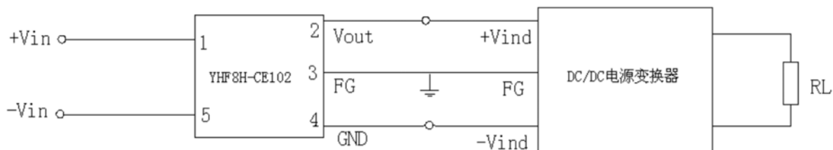
图 3 典型应用图
