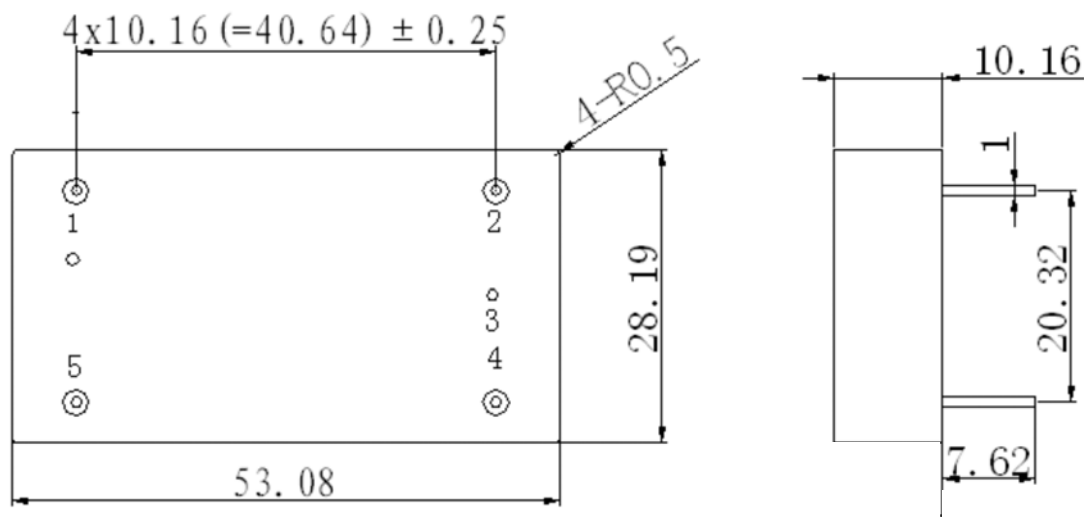
（7H 外形图 底视图）
