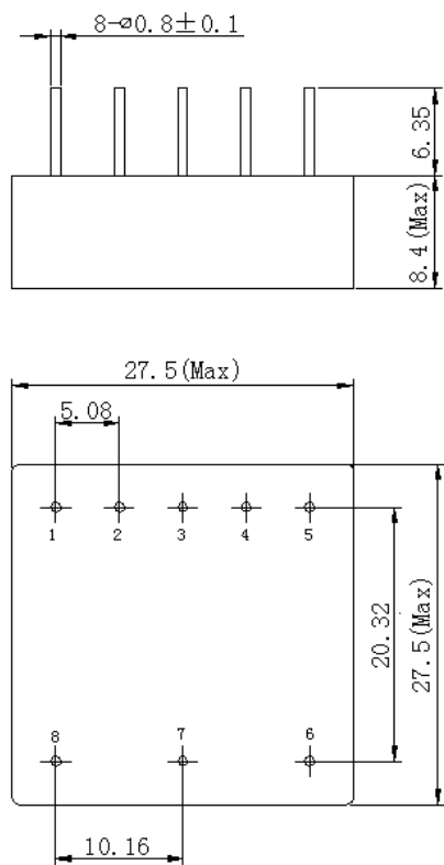
底视图
