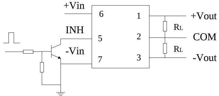
图 4 禁止端连接图
