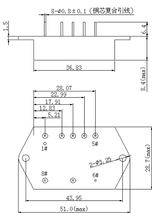
底视图
