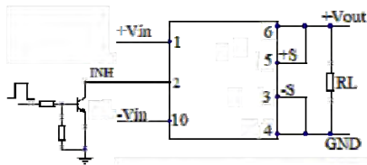
图 5 单路禁止端连接图
