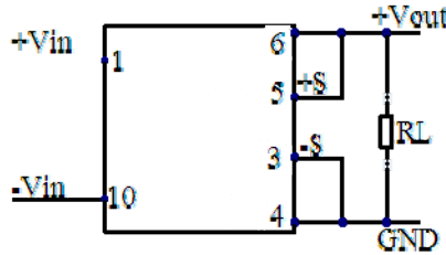
图 7 标称输出电压连接图
