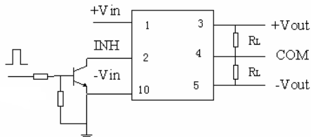
图 6 双路禁止端连接图
