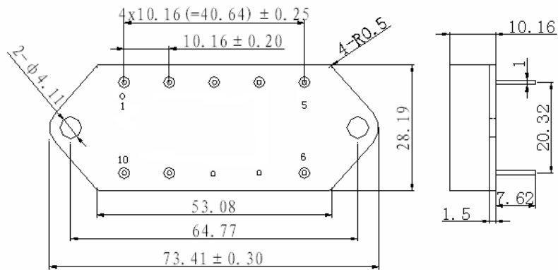
底视图
