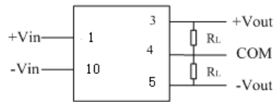
图 4 双路使用连接图
