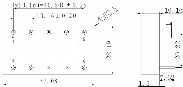
底视图
