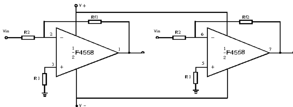
图 1 基本接线图
