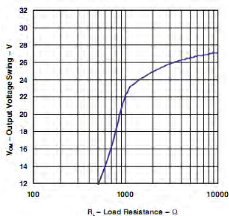
特性 3 输出幅度对负载电阻
