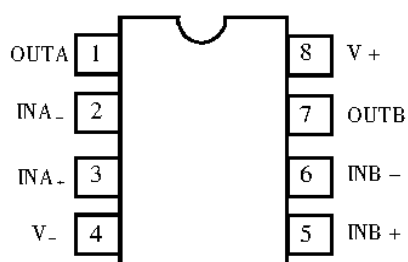
DIP、CSOP 型
