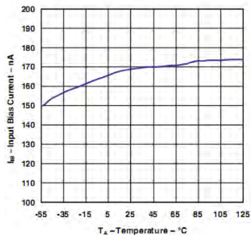
特性 2 输入偏置电流对温度
