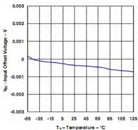
特性 1 输入失调电压对温度
