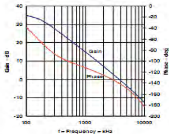
特性 4 开环电压增益对频率
