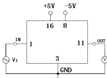
图 5 典型应用图
