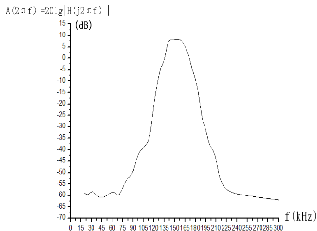
图 3 幅频特性曲线图
