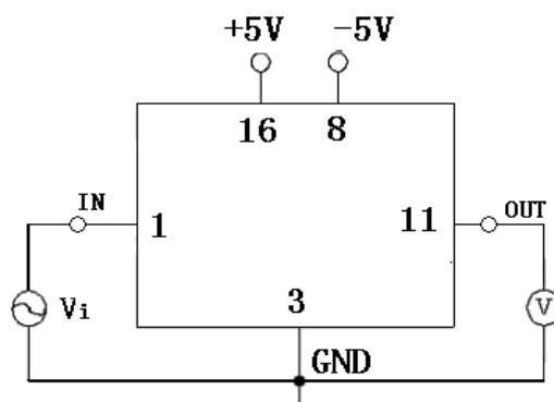
图 5 典型应用图
