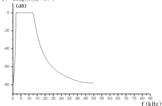
图 3 幅频特性曲线图
