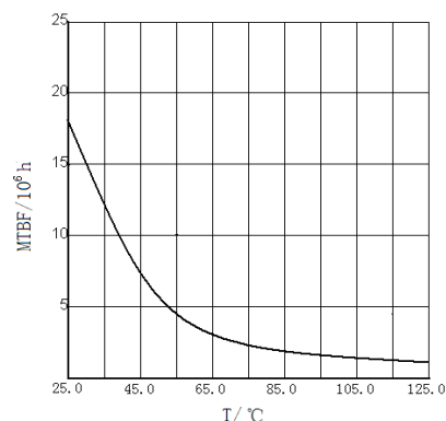
图 4 MTBF 温度曲线
