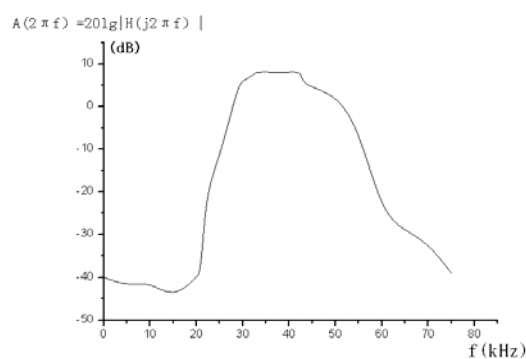
图 3 幅频特性曲线图
