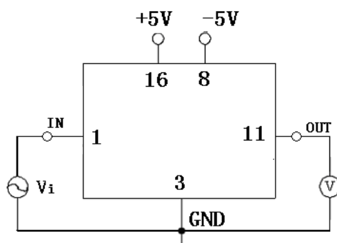
图 5 典型应用图
