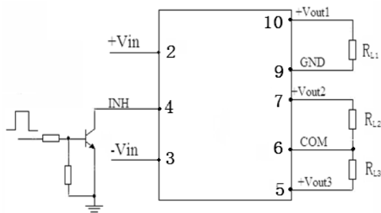
图 4 禁止端连接图
