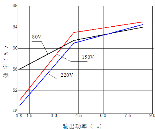
图 2 YH6T9-70/220S5S12S5 效率 (输出功率)
