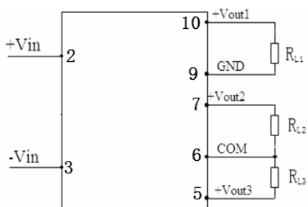
图 3 使用连接图
