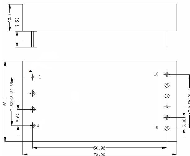
底视图 图 1 外形尺寸
