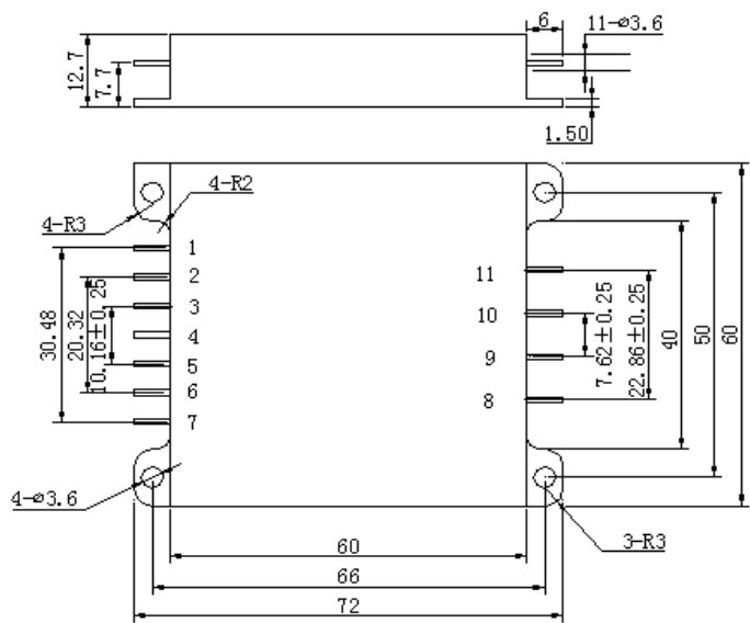
图 1 外形尺寸
