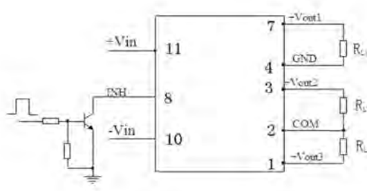
图 4 禁止端连接图
