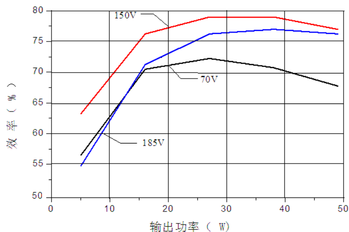
图 2 YH719 效率（输出功率）
