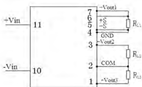
图 3 使用连接图
