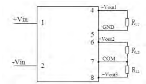
图 3 使用连接图
