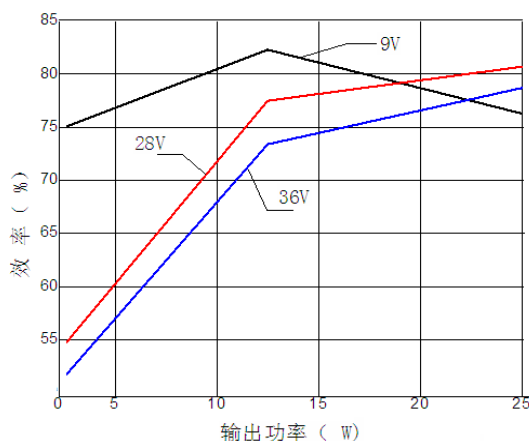
图 2 YH717 效率（输出功率）
