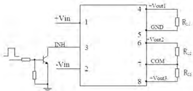
图 4 禁止端连接图
