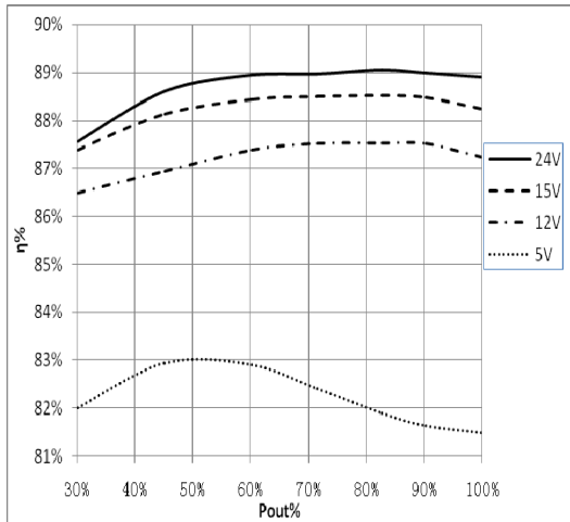
110V (66V~154V) 输入模块输出功率-效率曲线 输出电压: 5V, 12V, 15V, 24V
