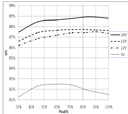
300V (180V~375V) 输入模块输出功率-效率曲线 输出电压为: 5V, 12V, 15V, 24V
