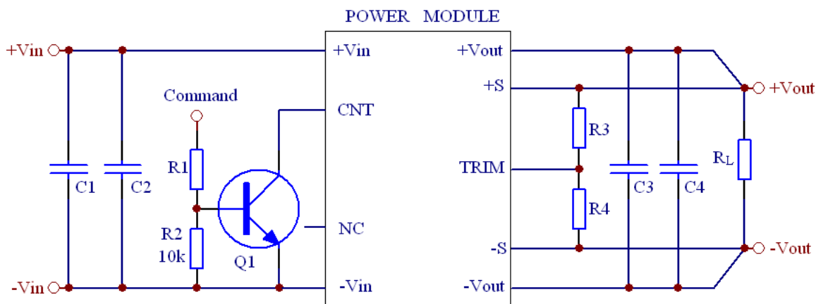
图 1 模块应用电路图
